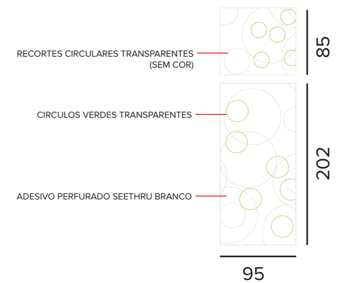
PORTA CONCILIAÇÃO - 1 FOLHA
