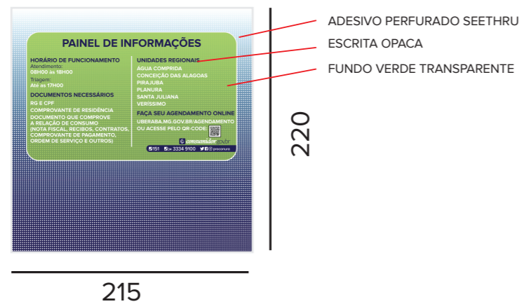
PORTA AUDITÓRIO - 2 FOLHAS
